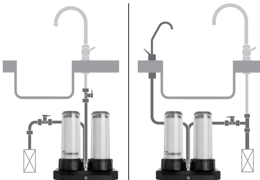
Einbauschema DUO Classic
